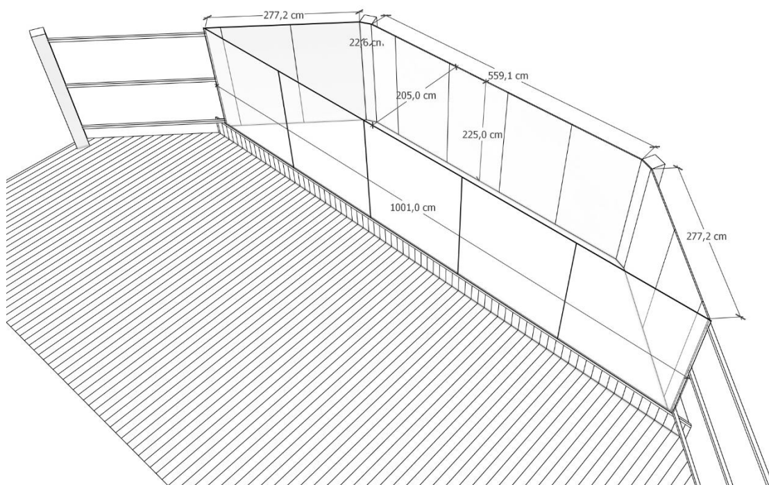
Rys. 1 – Schemat części sceny przeznaczonej pod ekspozycję
